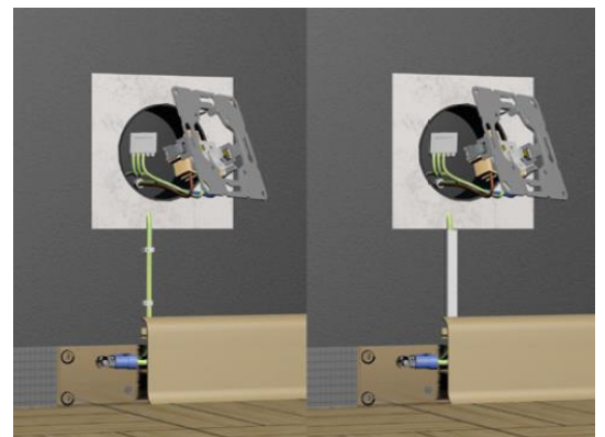
Abb.3 Erdungsdraht sichtbar / Erdungsdraht in Kanal verlegt / Einführen des Erdungsdrahtes in die Wanddose.
