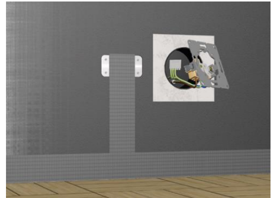
Abb.2 Erdungsplatte neben Steckdose / Führung des Erdungsbandes / Einführen des Erdungsdrahtes in die Wanddose.
