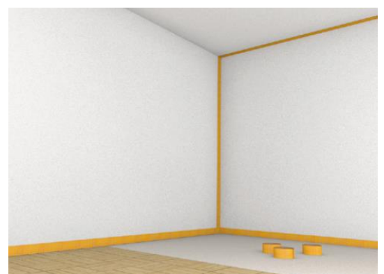
Abb.4 Aufkleben des elektrisch leitfähigen Erdungsbandes AEB im Sockelbereich. Soll der Deckenbereich geschirmt werden, wird das Erdungsband nach oben geführt und über die gesamte Deckenbreite verklebt.
